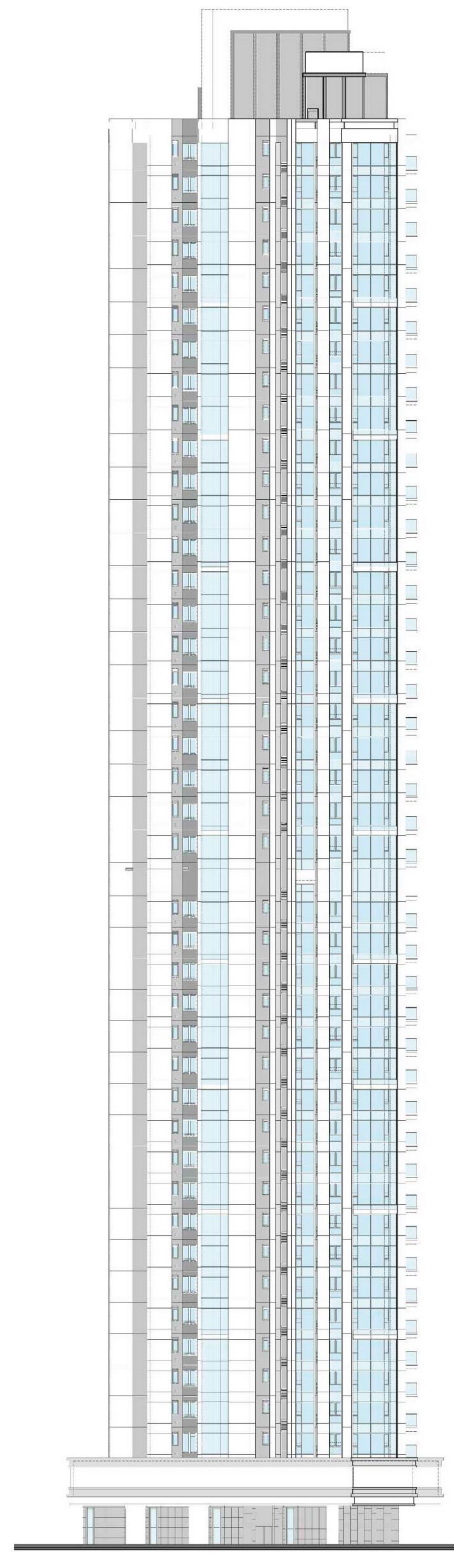
Elevation 12 立面 12
