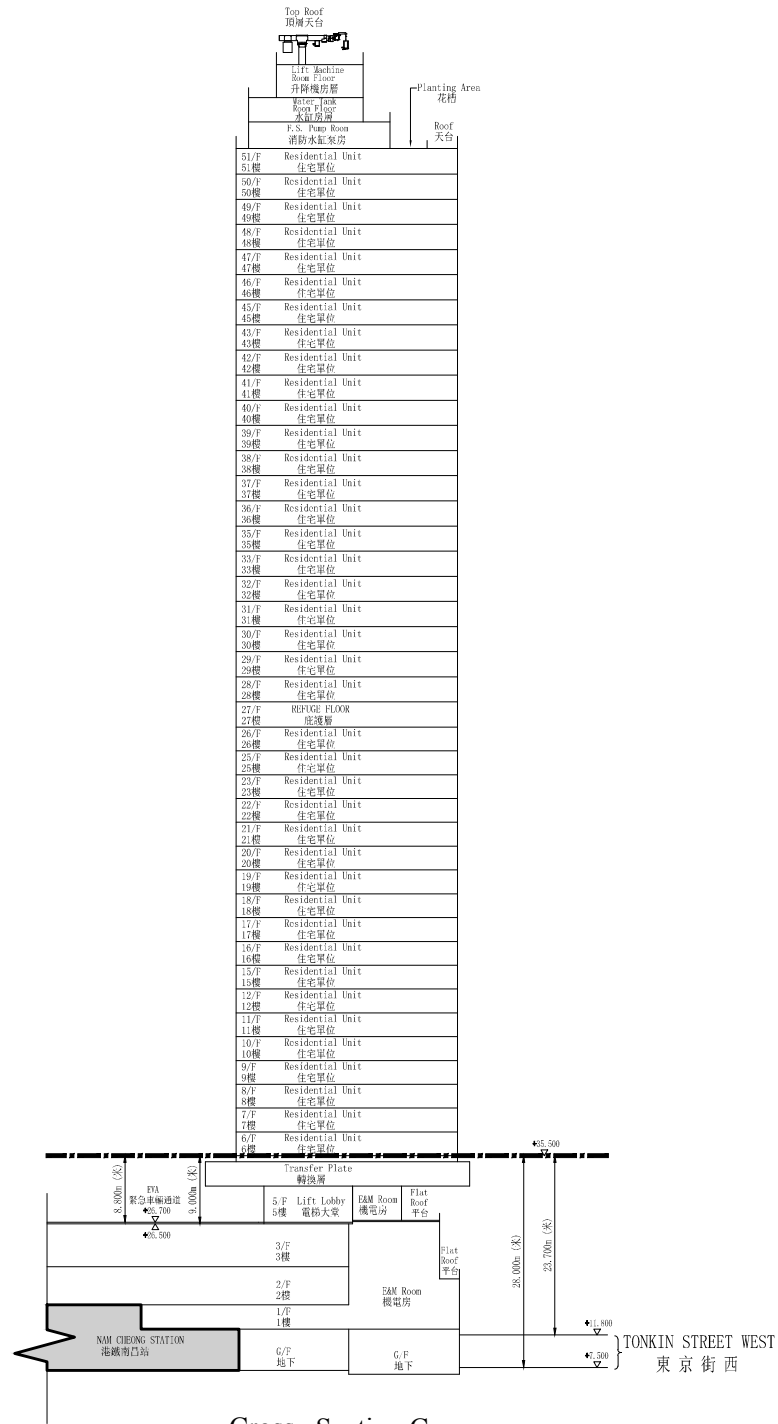
Cross - Section C 橫截面 C
